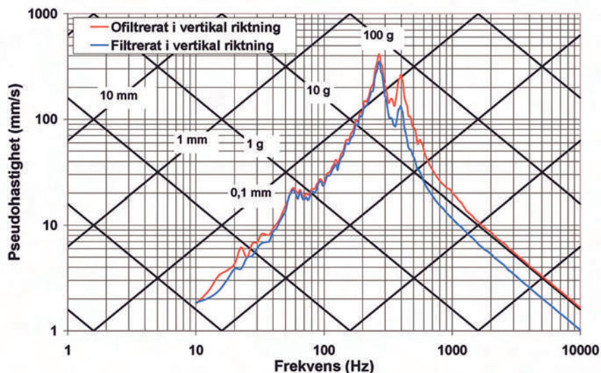
Figur 5: Responsspektrum av svängningsförloppet för en ofiltrerad och en filtrerad vibrationssignal, jämför figur 3 (responsspektrat är beräknat vid tre procent dämpning).
